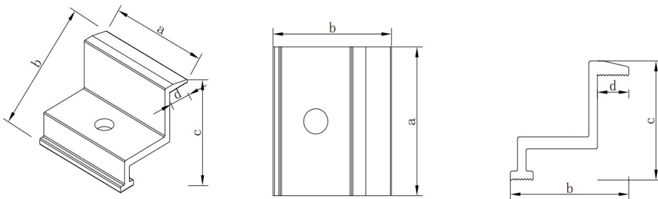
Fig. 5 Clamp
